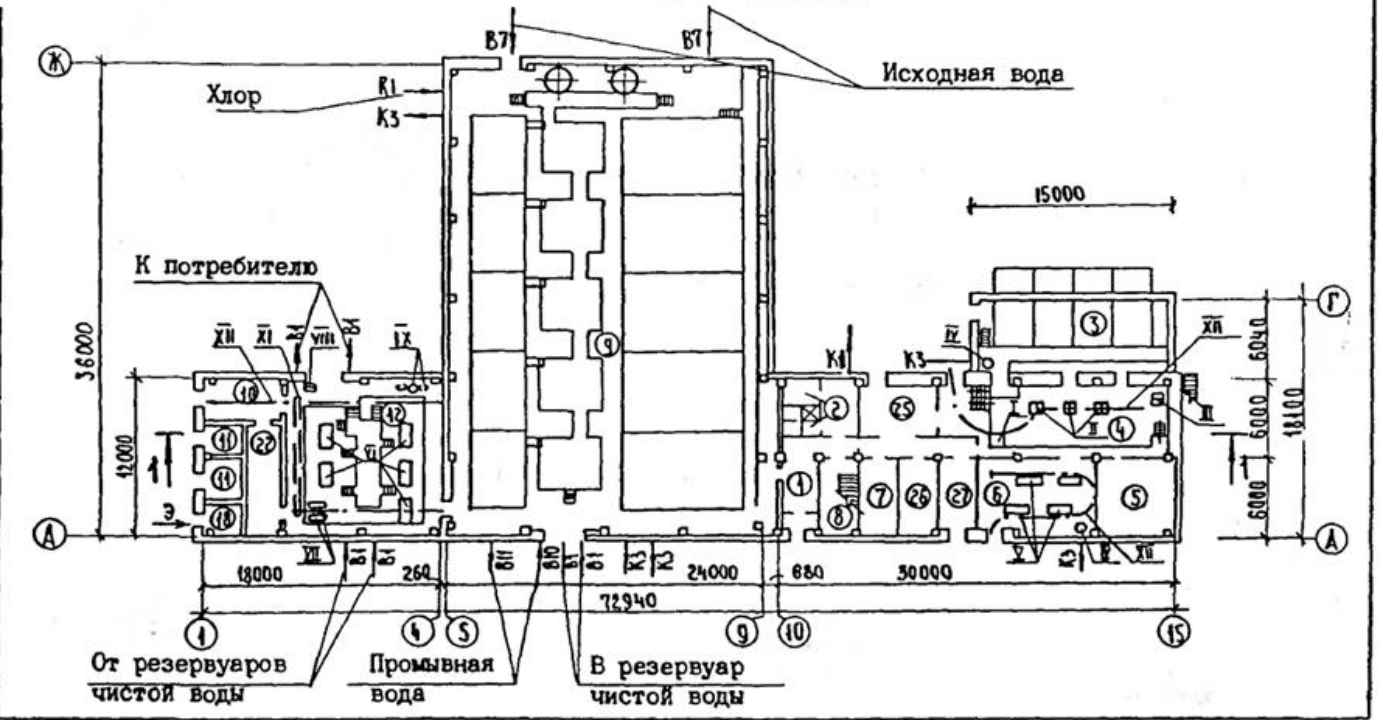
ПЛАН НА ОТМ. -2.400; -1.200, 0.000
