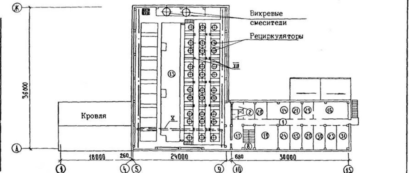
ПЛАН НА ОТМ. -2.400; -1.200, 0.000
